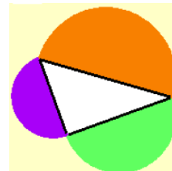
Generalización utilizando figuras semejantes sobre los lados del triángulo.
