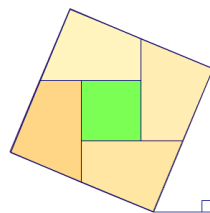
Construcción de Henry Perregal, Matemático inglés (1801-1898)
