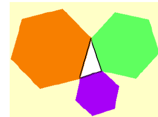
Generalización utilizando figuras semejantes sobre los lados del triángulo.
