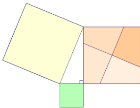
Construcción de Henry Perregal, Matemático inglés (1801-1898)
